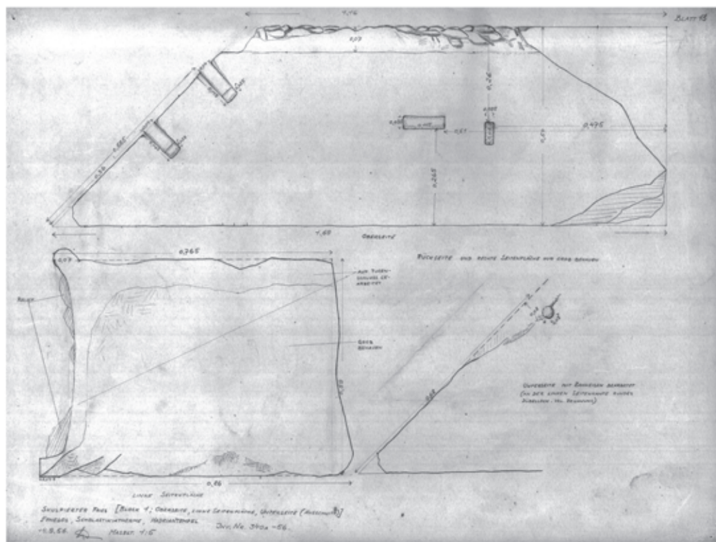
2 Relief, Ephesos Museum Selçuk Inv. 713, Draufsicht, linke Seitenfläche Unteransicht, Zeichnung K. H. Göschl
