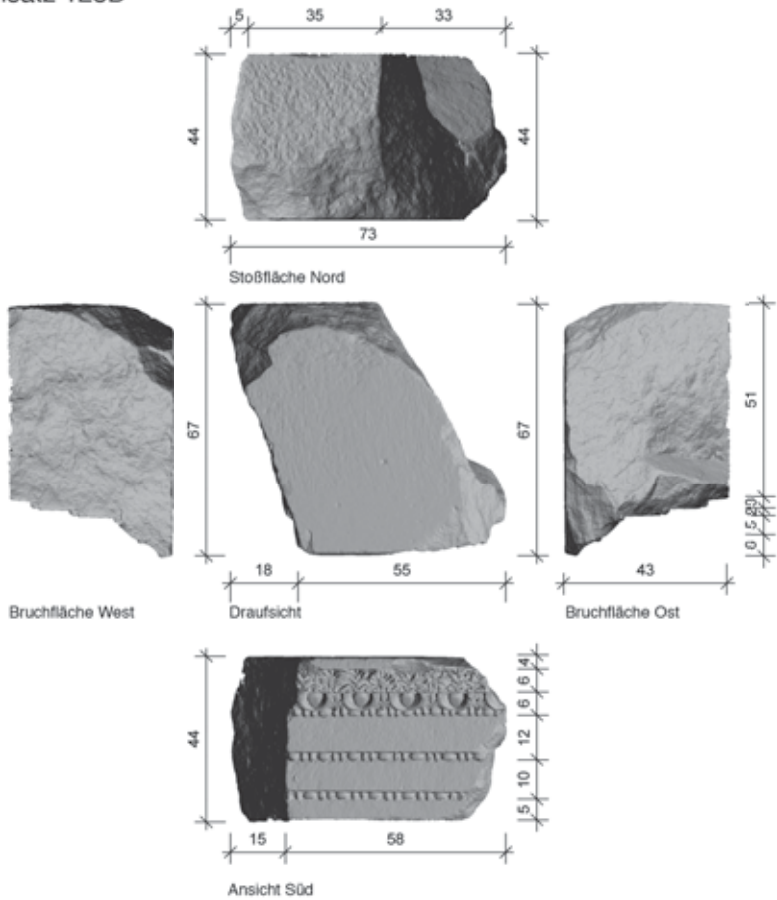
Architrav 123A Gurtbogenansatz 128D
