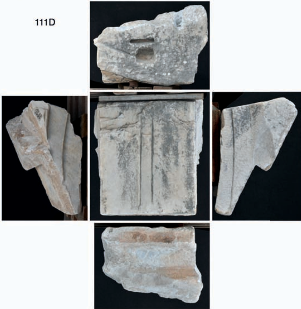
Gurtbogenansatz 111D. 112D
